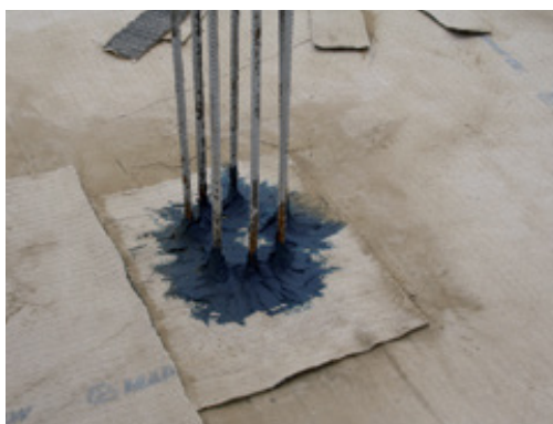
Vytesnenie dodatočného bentonitového pásu Mapeproof okolo ocelevej výstuže s použitím Mapeproof Mastic
